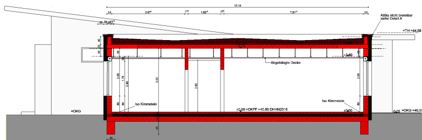
SNITT A-A'
